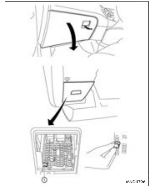
Hauptsicherungskasten Rechtslenker
